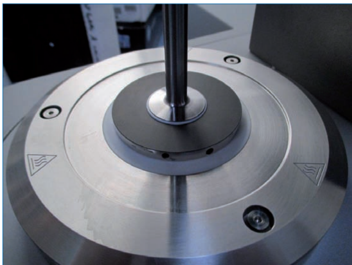
Bild 1: Messspalt des MCR 302
